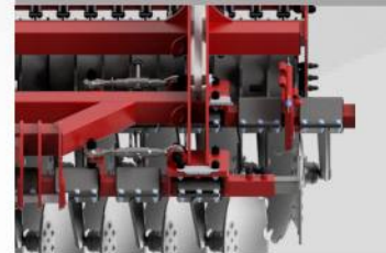
Verstellbare Scheibenreihen
